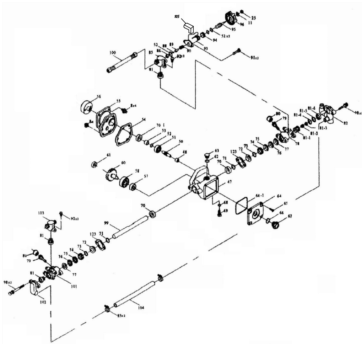
3WZ-6F背负式动力喷雾机分解图(2)
