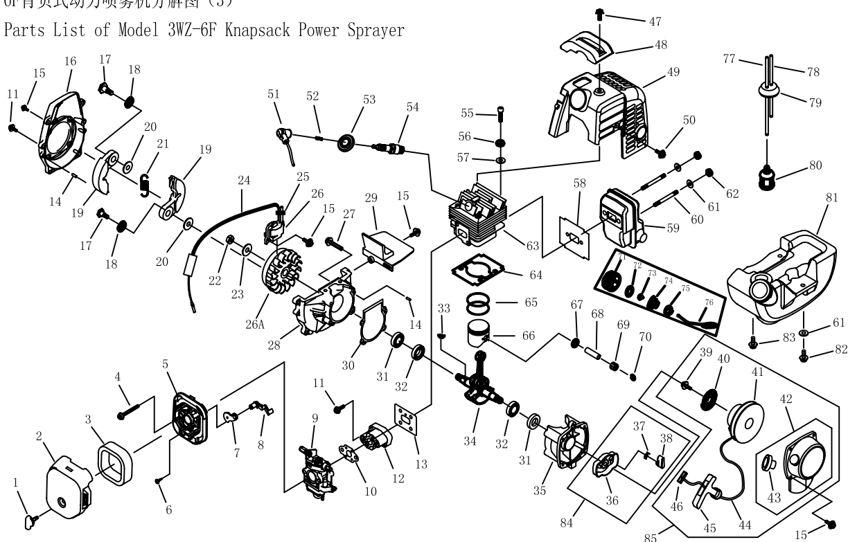
3WZ-6F背负式动力喷雾机分解图 (3)
